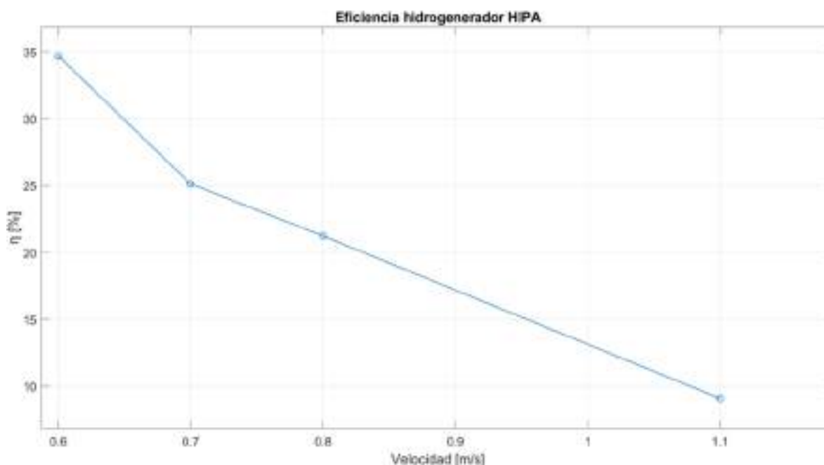
Figura 5 Eficiencia a diferentes velocidades de la corriente
